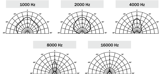
Corneta CHL 14-25 Trinyum acoplada ao driver HDT 600 em câmara anecóica (1 W / 1 m).
