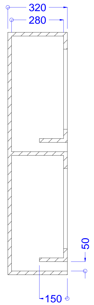
Seção A-A
