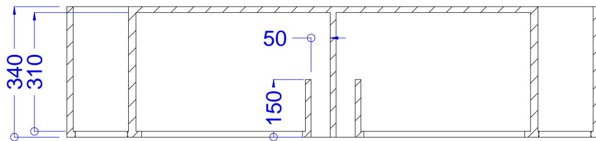
Seção B-B
