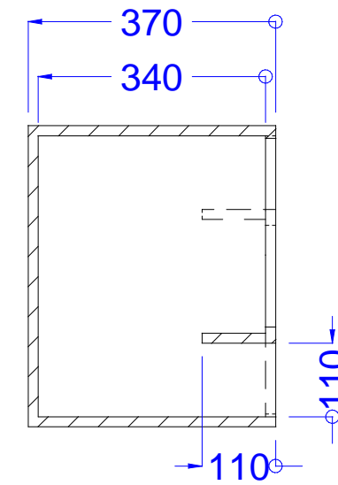
Seção B-B
