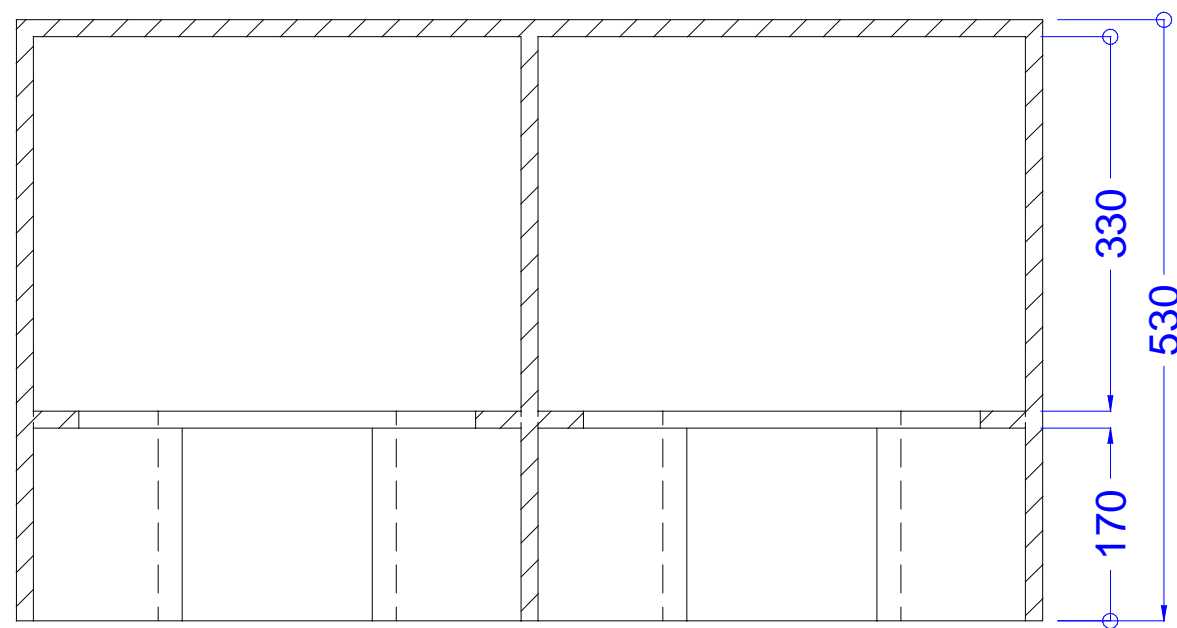
Seção A-A
